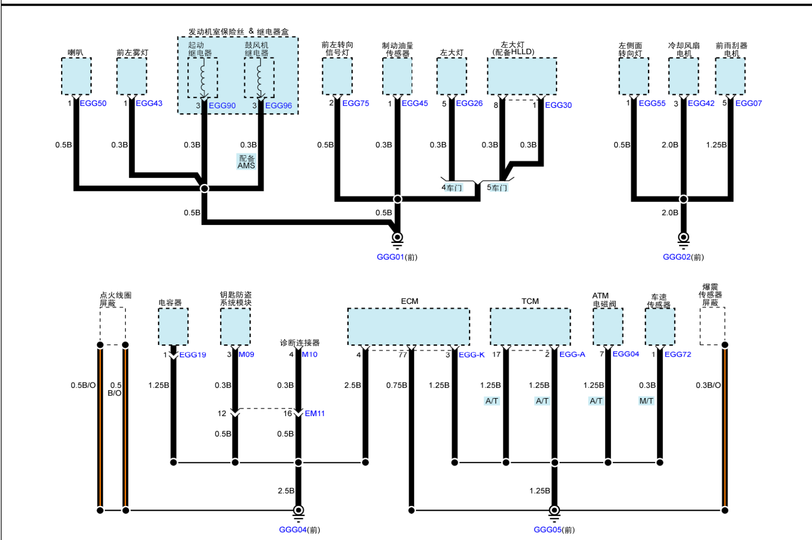
搭铁分布 (6)
