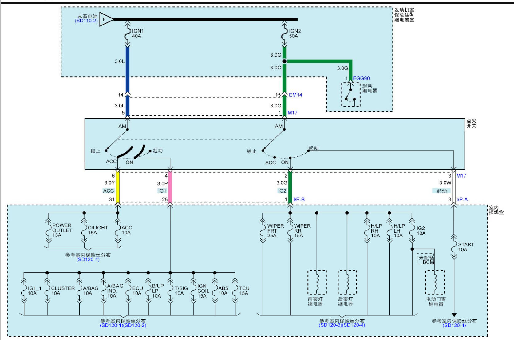
电源分布 (3)
