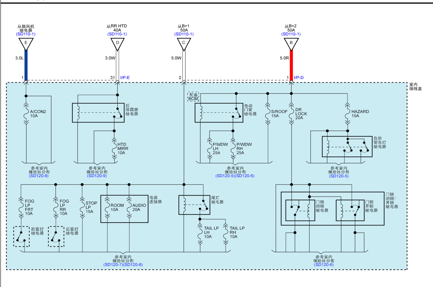
电源分布 (4)
