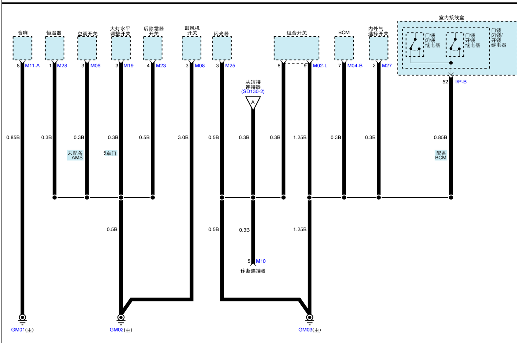
搭铁分布 (1)
