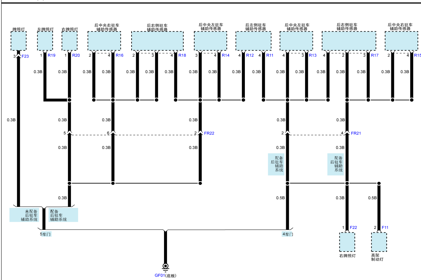
搭铁分布 (3)
