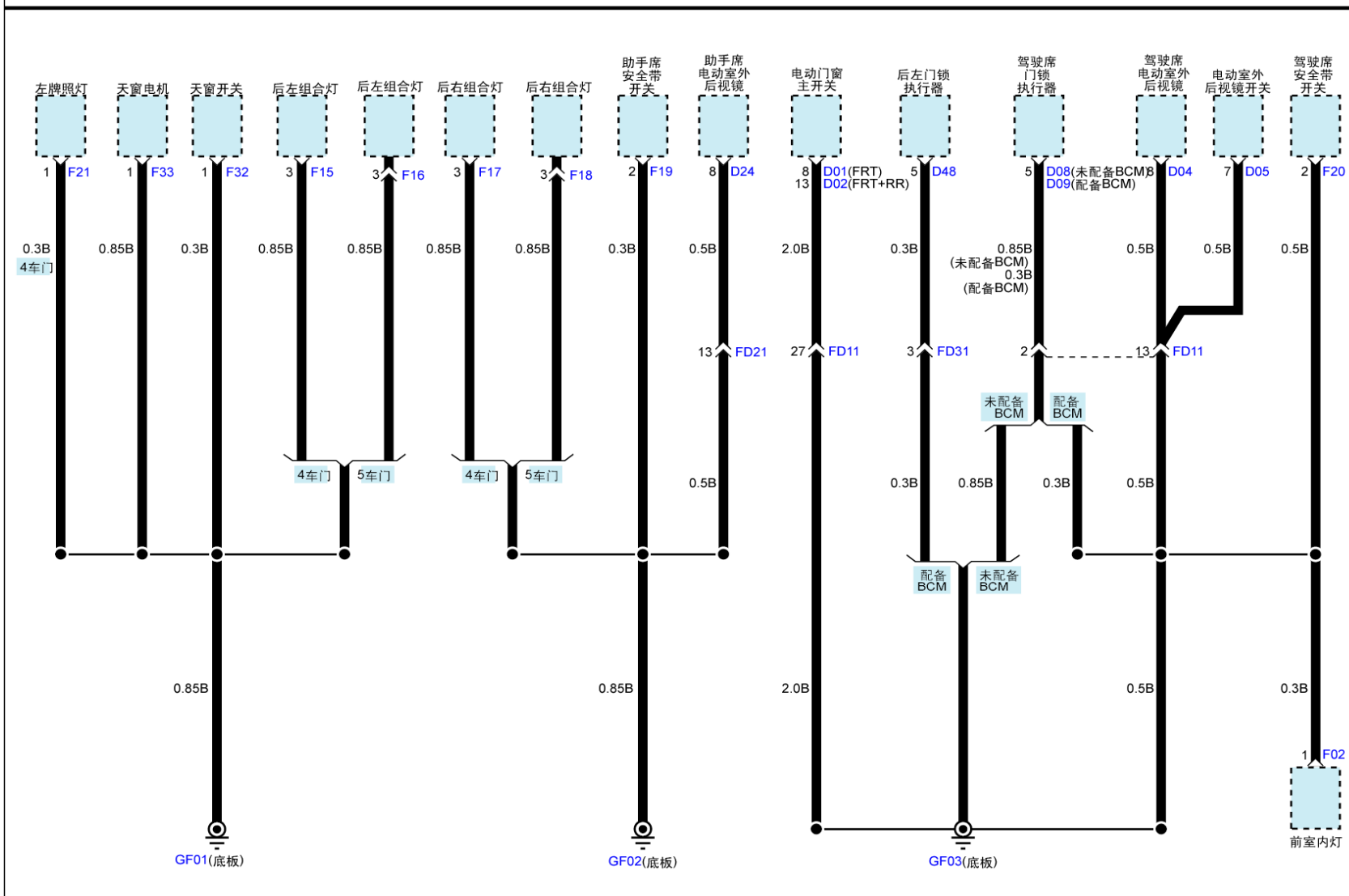
搭铁分布 (4)
