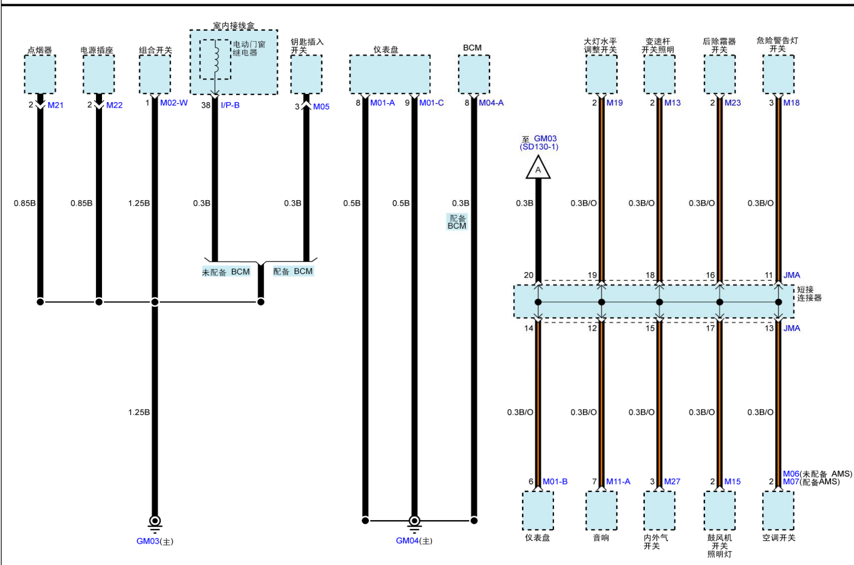
搭铁分布 (2)
