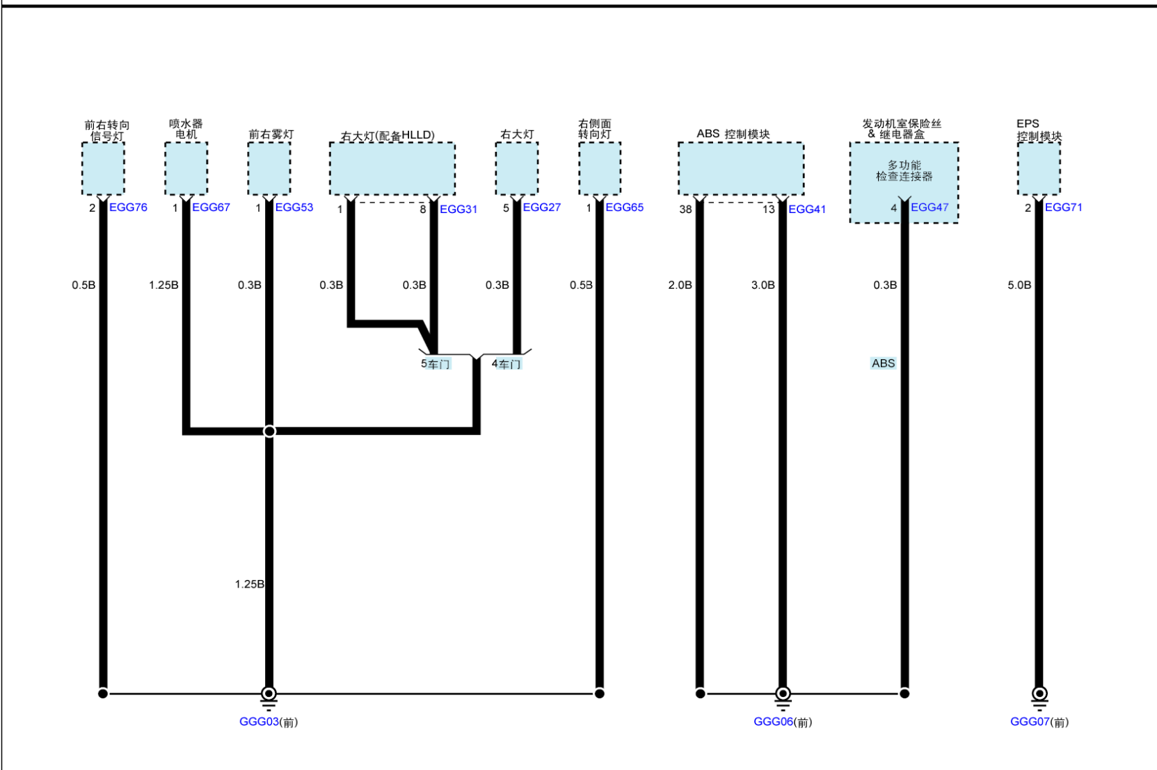
搭铁分布 (7)
