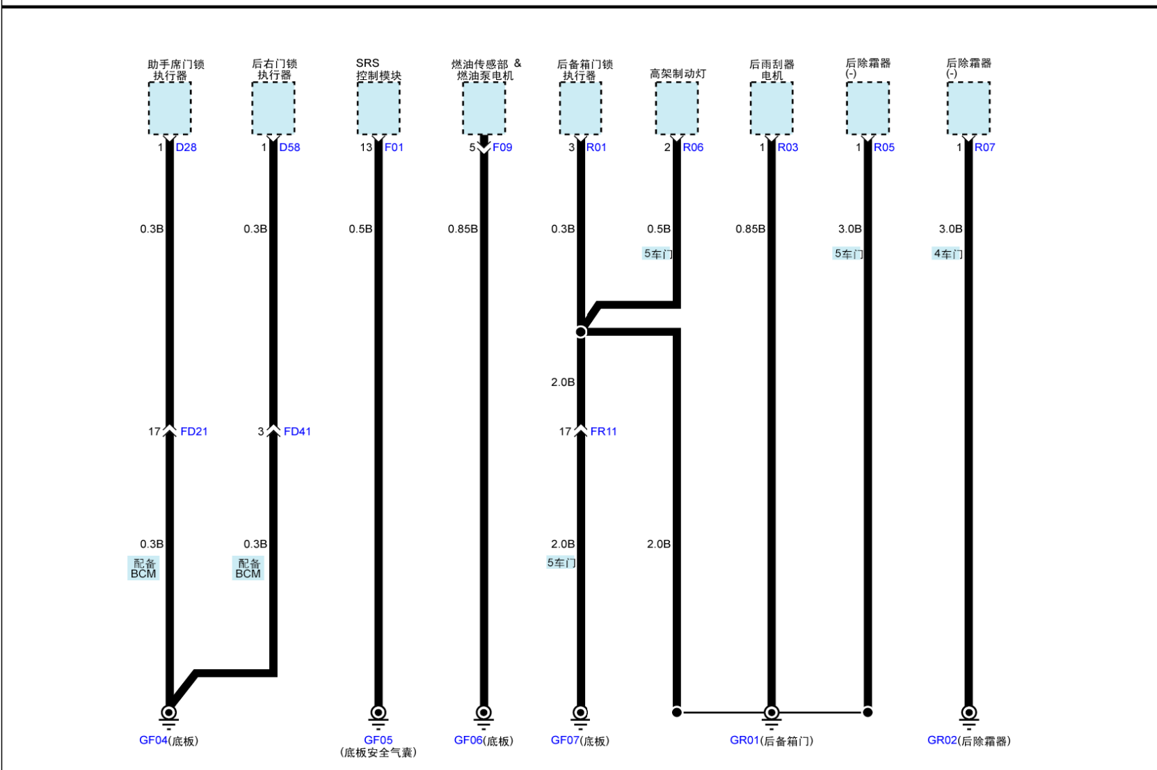
搭铁分布 (5)
